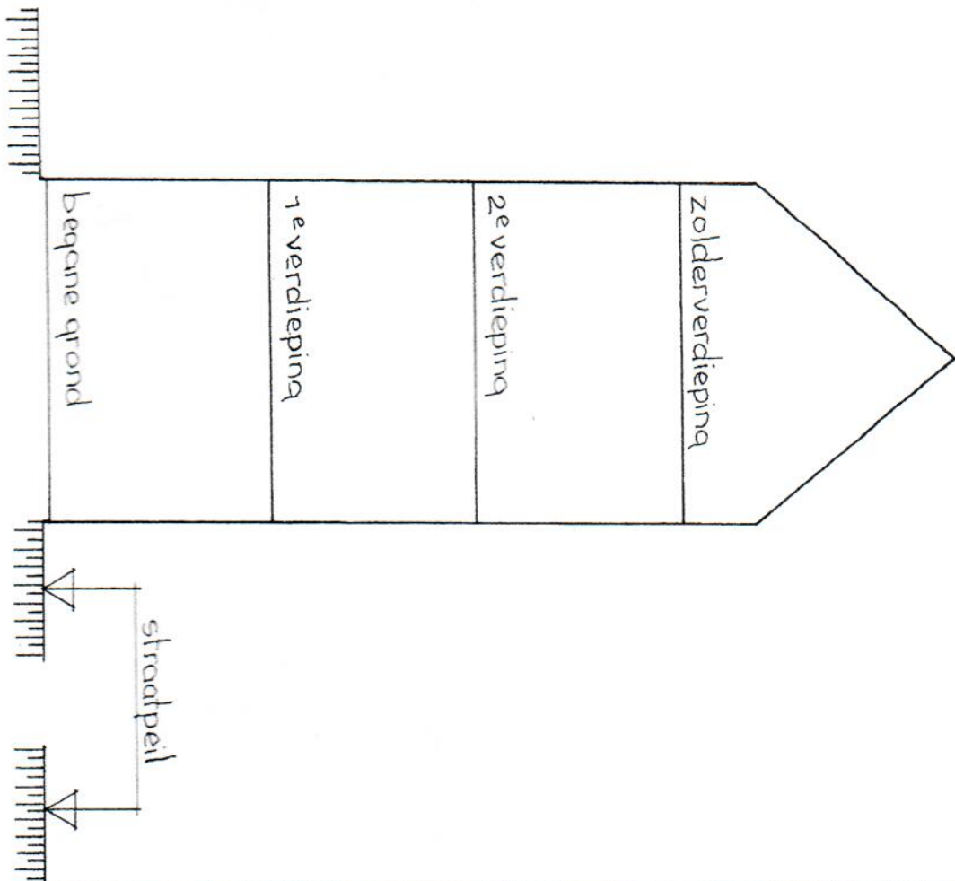
Dwarsdoorsnede 1:100
